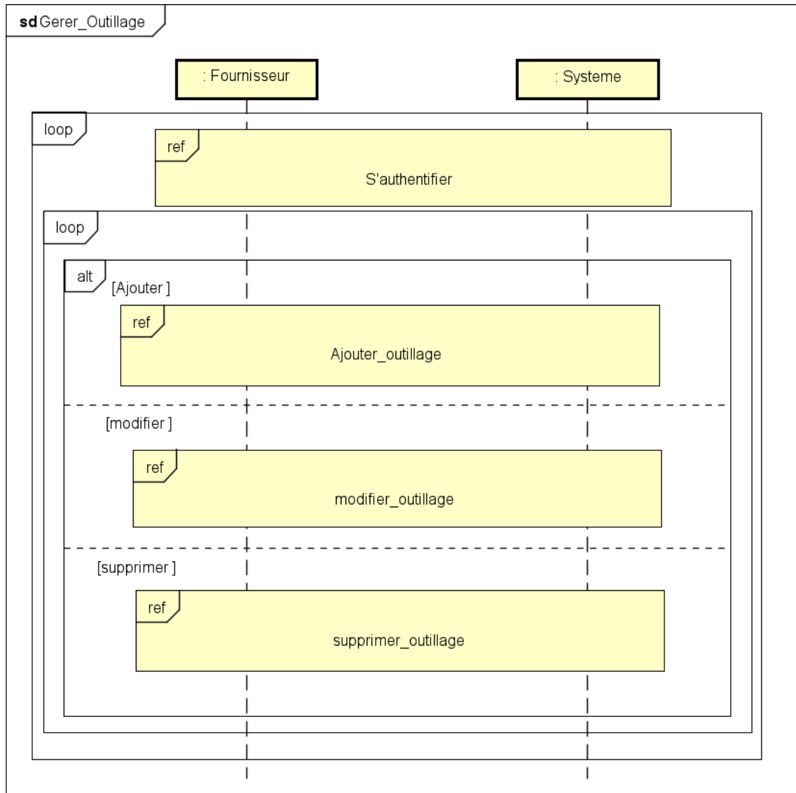
Figure 64 Diagramme de séquence de gérer outillage
