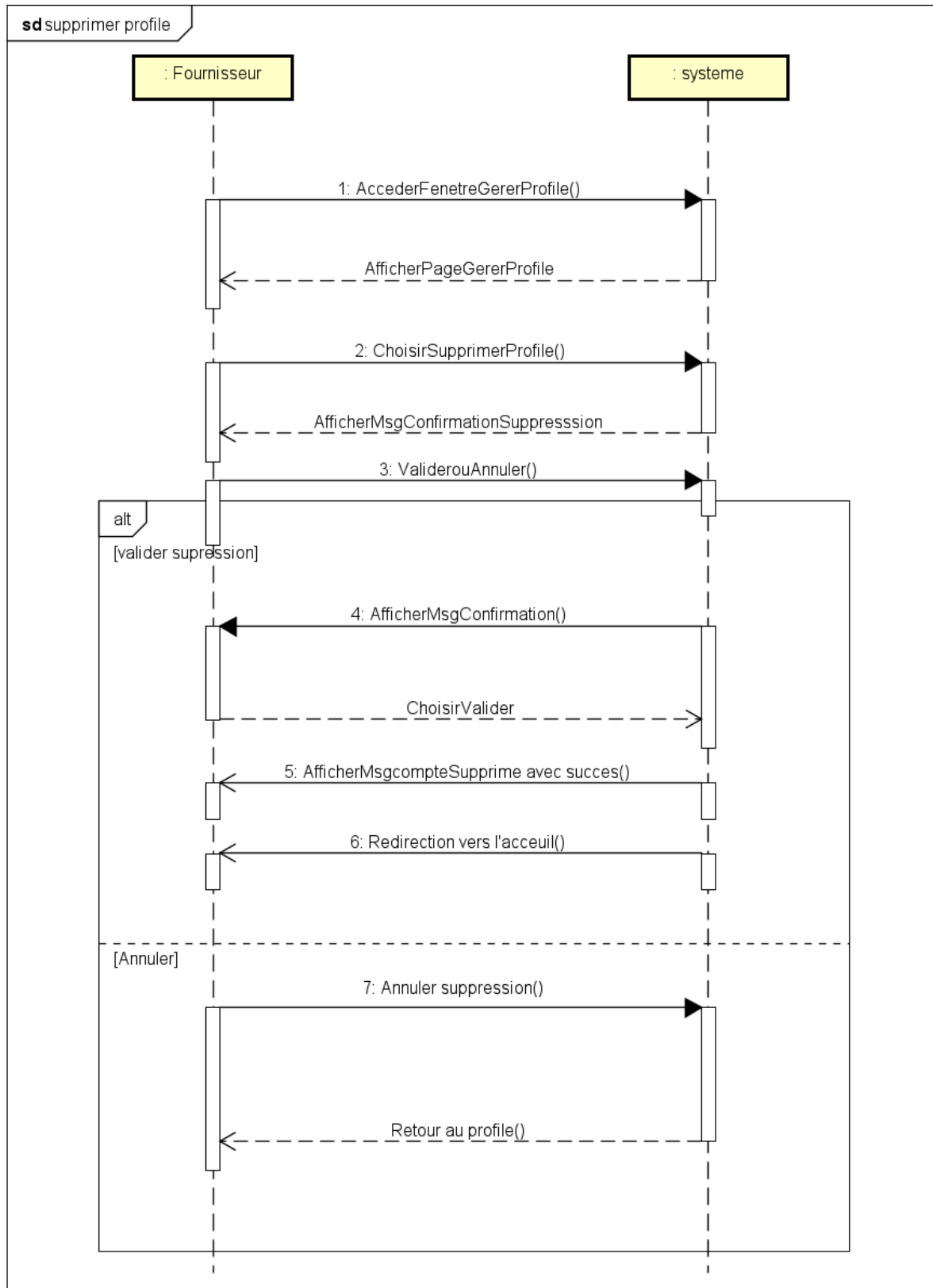
Figure 58 Diagramme de séquence de supprimer profile
