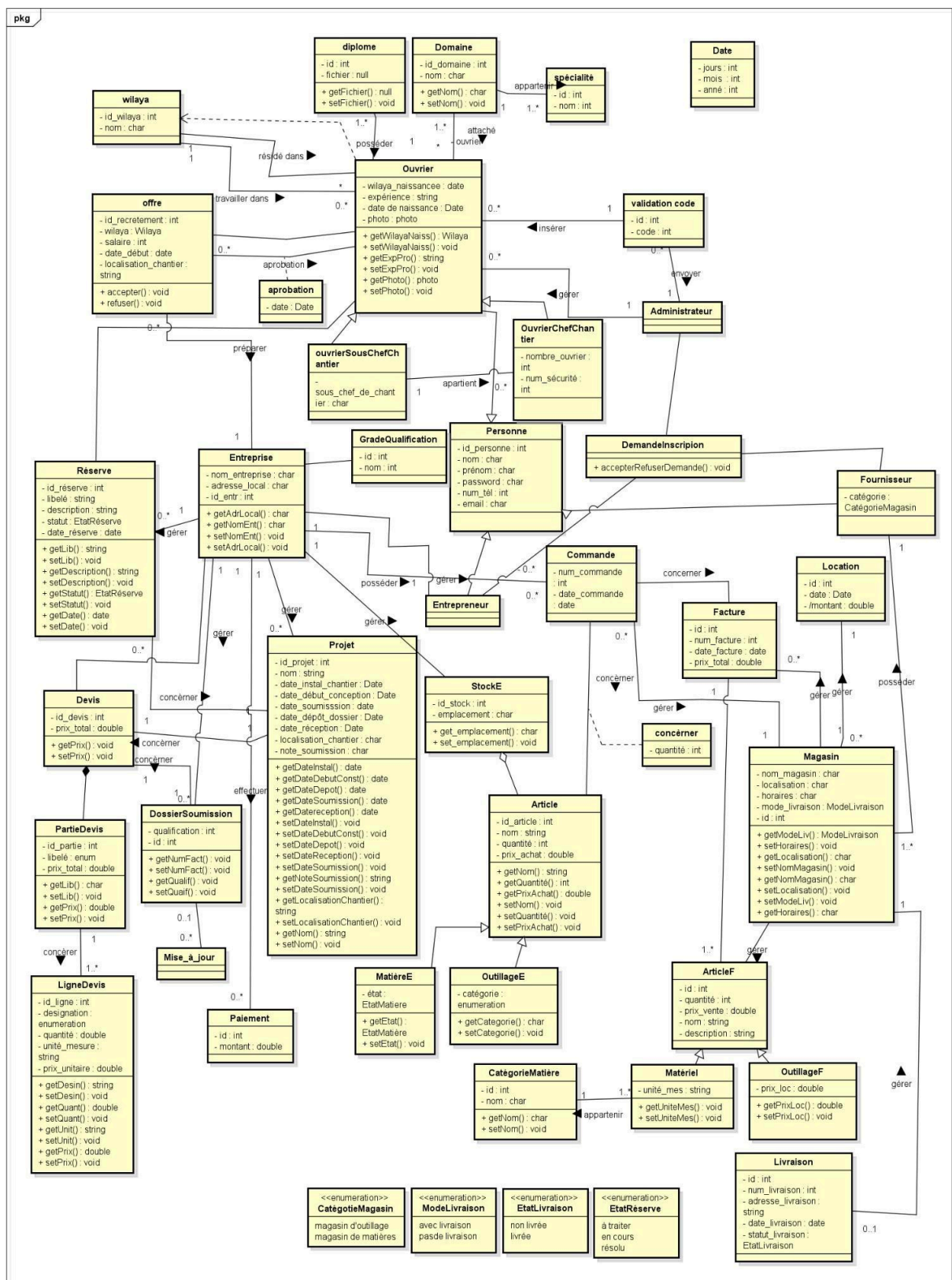
Figure 14 Diagramme de classe d'analyse
