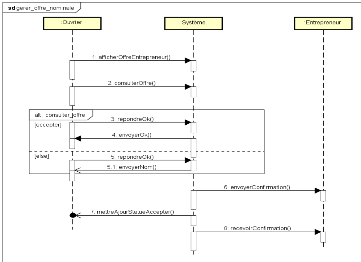
Figure 92 Diagramme de séquence de gérer offre
