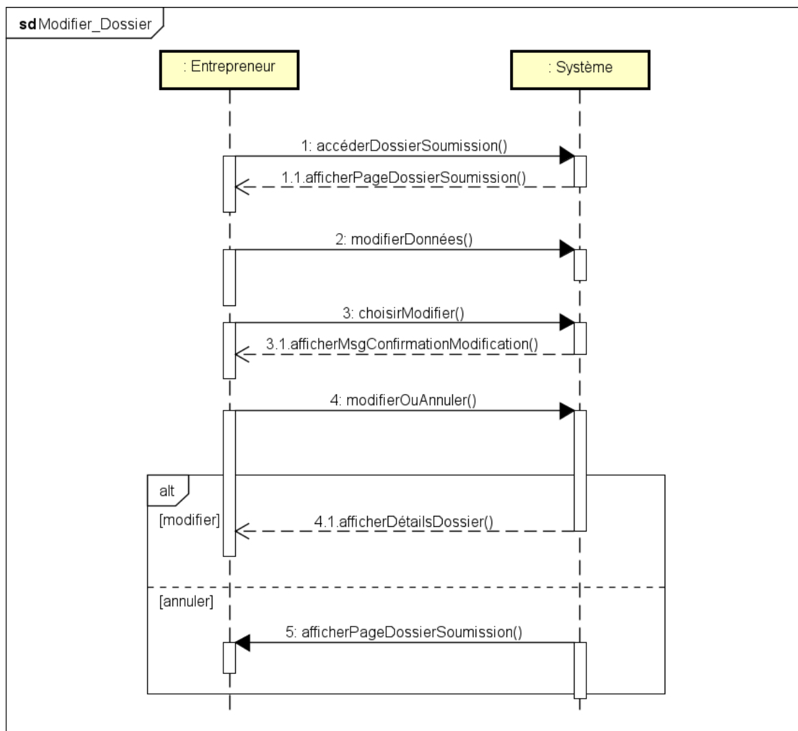
Figure 44 Diagramme de séquence de modifier dossier de soumission
