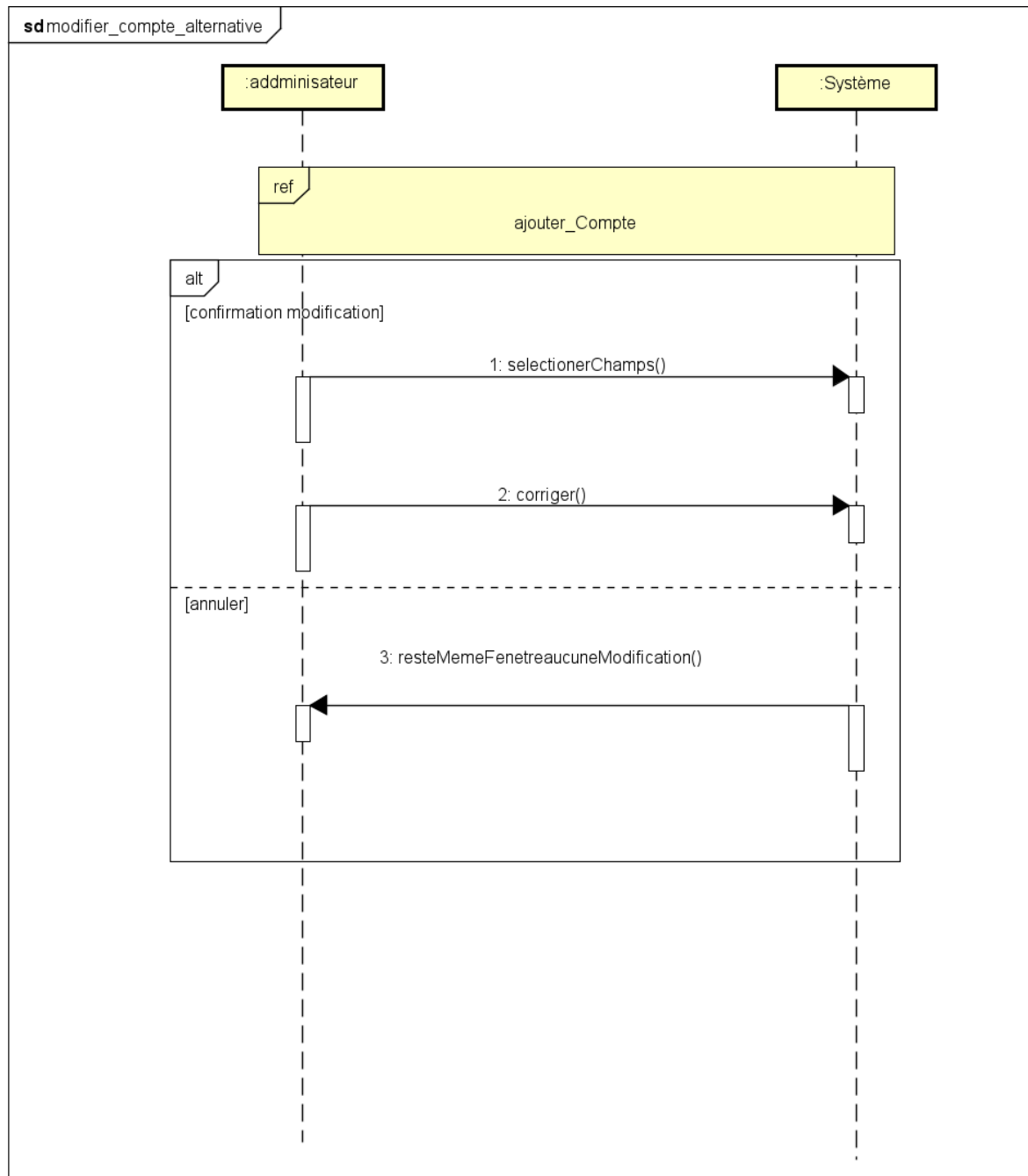
Figure 96 Diagramme de séquence de modifier compte alternatif
