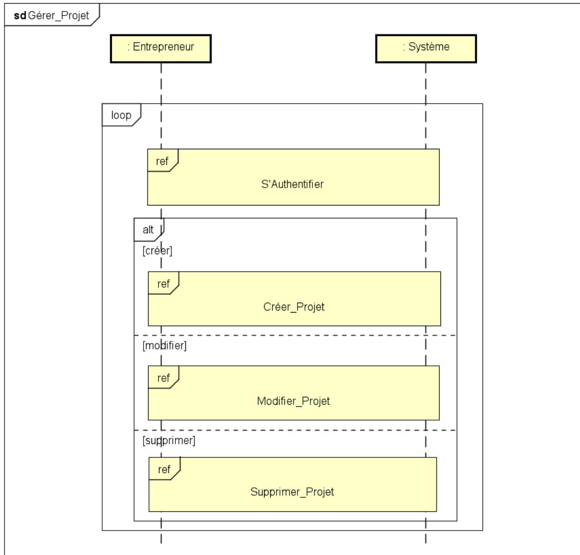
Figure 45 Diagramme de séquence de gérer projet
