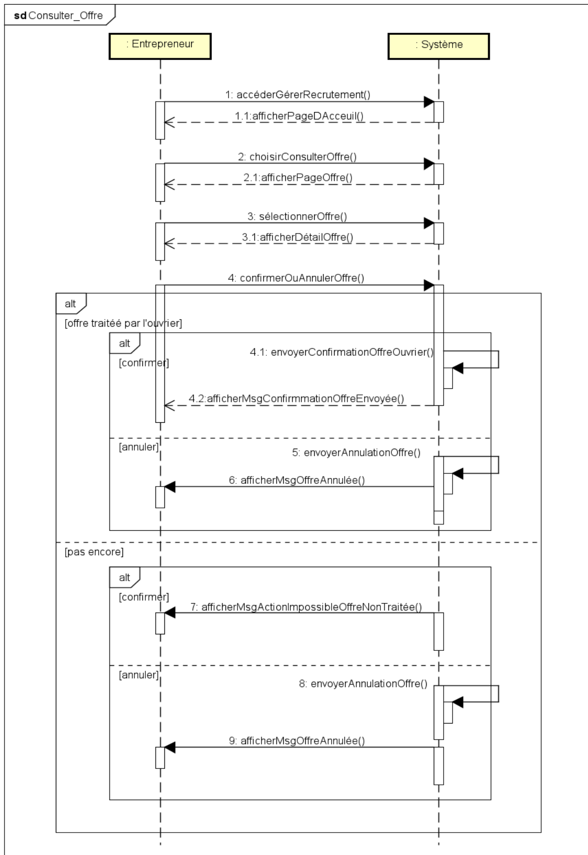
Figure 33 Diagramme de séquence de consulter offre
