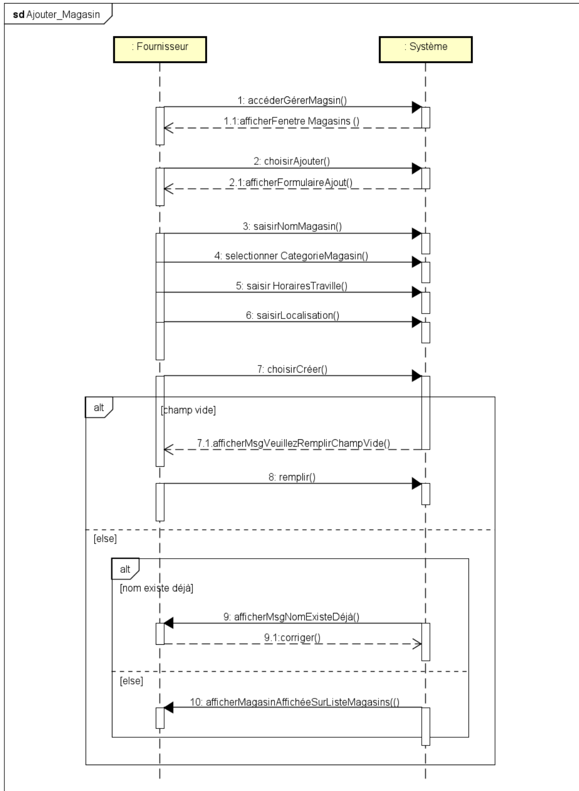
Figure 68 Diagramme de séquence ajouter magasin
