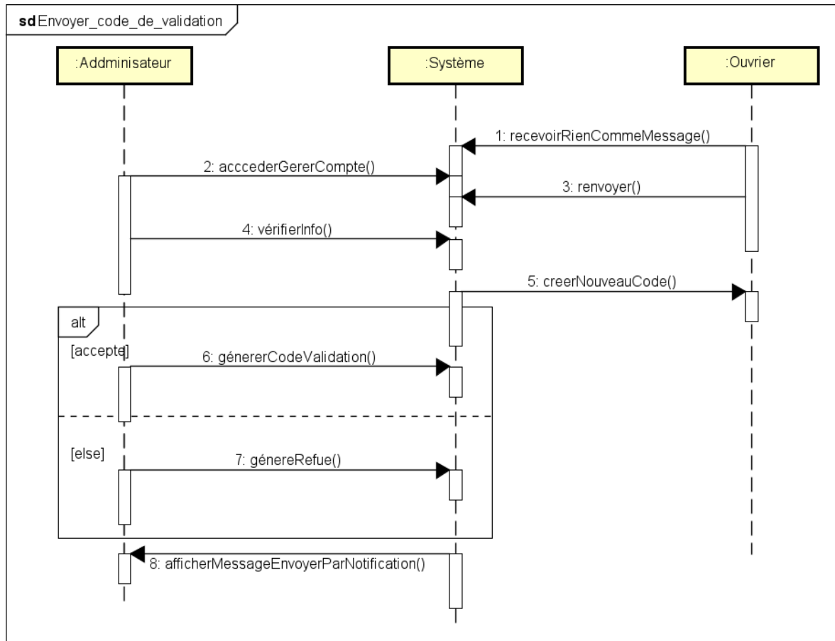
Figure 99 Diagramme de séquence d' envoyer code de validation
