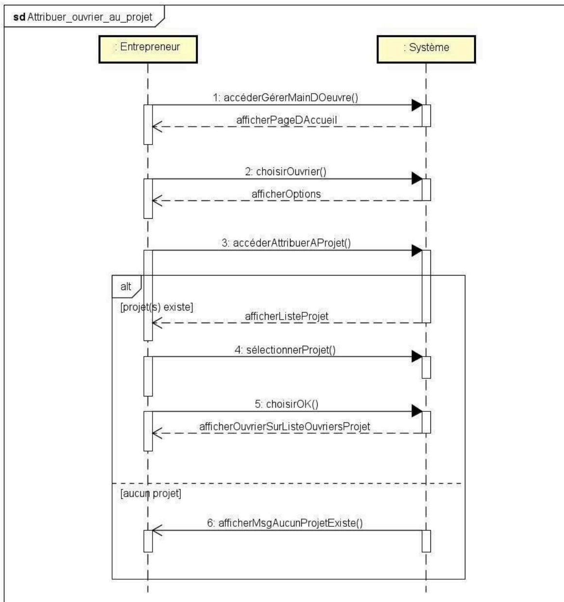
Figure 32 Diagramme de séquence d'attribuer ouvrier au projet
