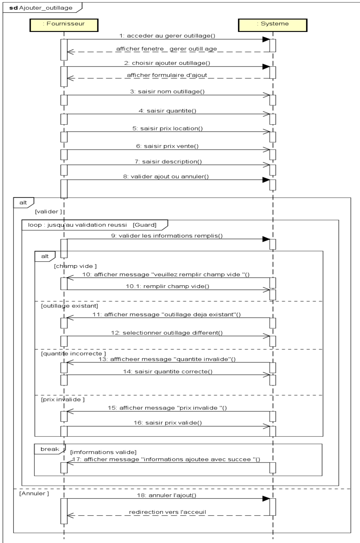
Figure 65 Diagramme de séquence d'ajouter outillage
