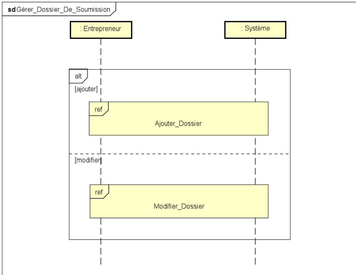
Figure 42 Diagramme de séquence de gérer dossier de soumission
