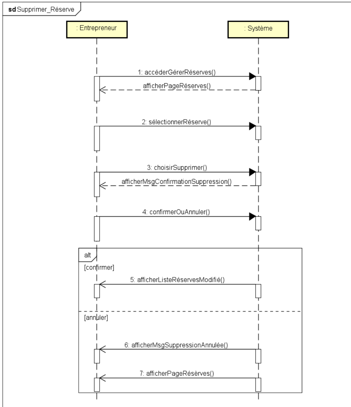
Figure 41 Diagramme de séquence de supprimer réserve
