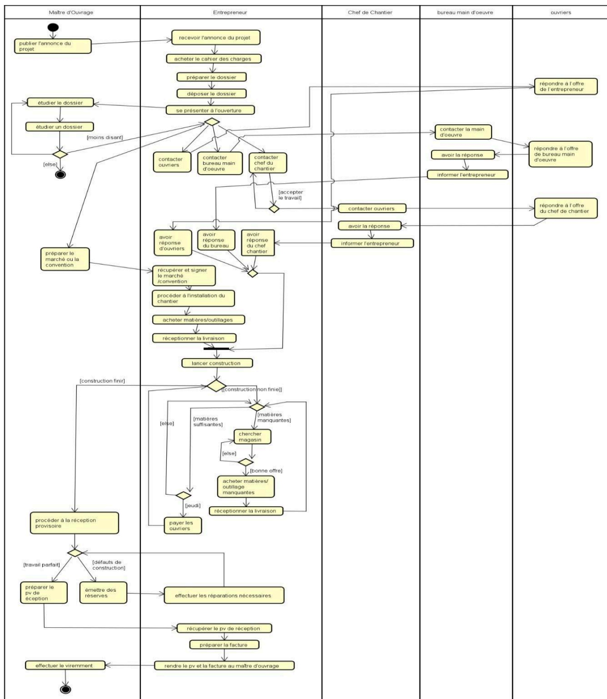
Figure 1 Diagramme d'activité du processus métier d'entrepreneur
