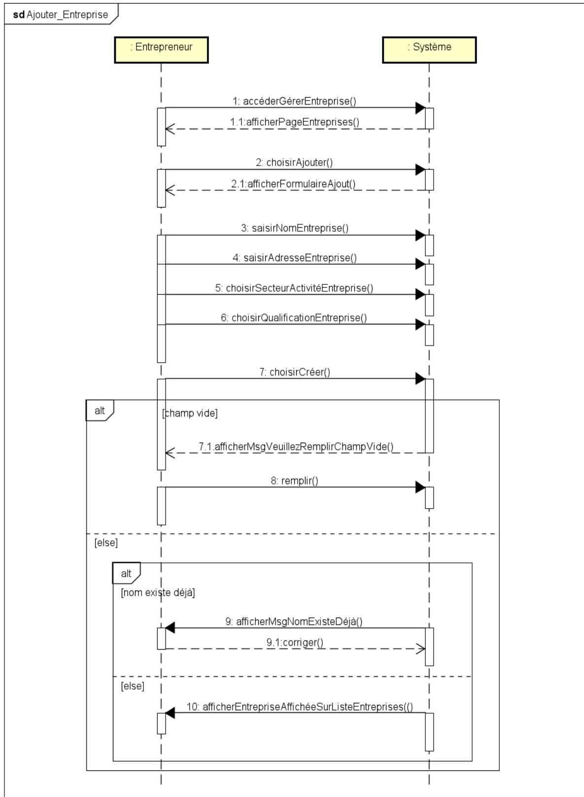
Figure 50 Diagramme de séquence de d'ajouter entreprise
