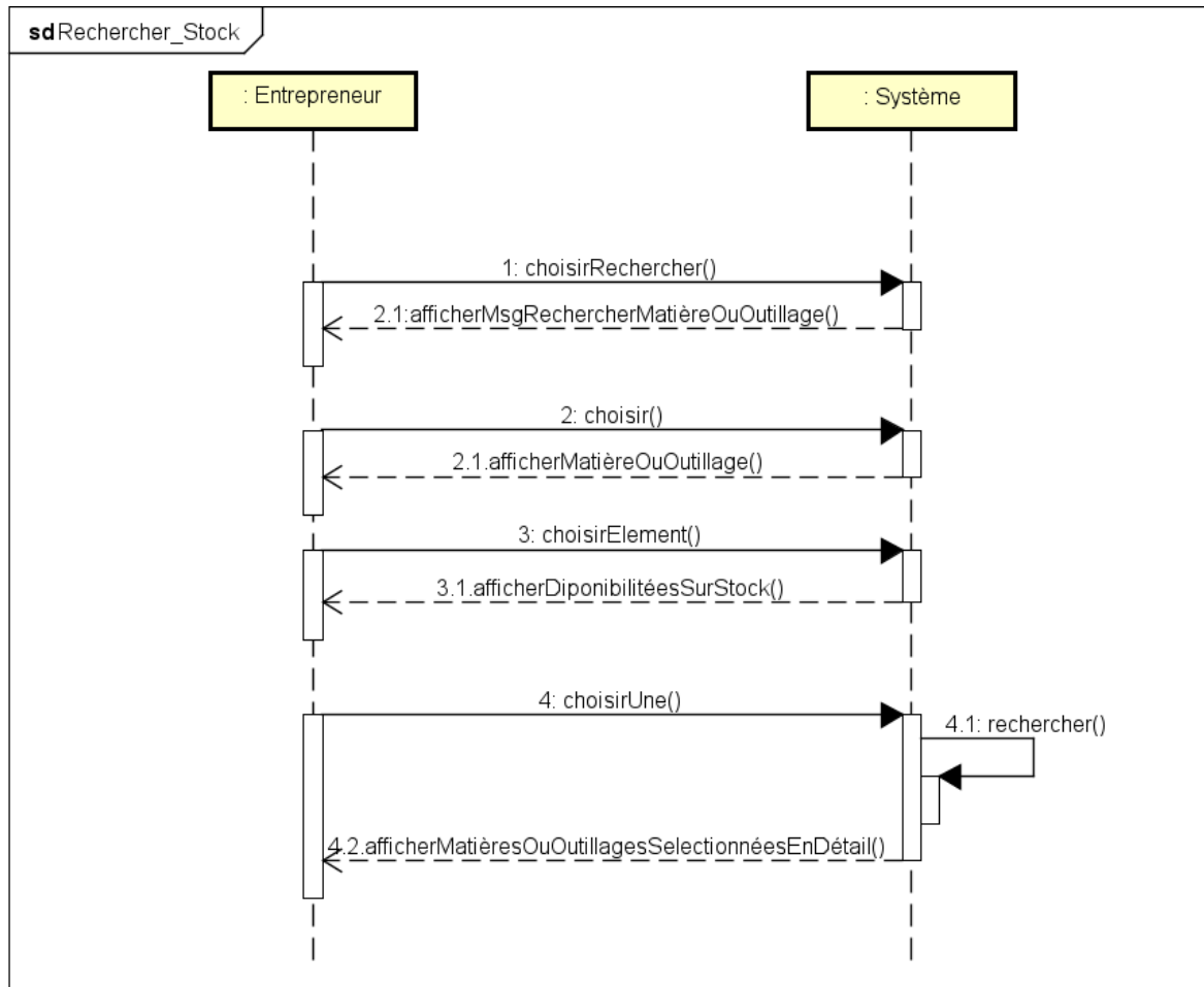
Figure 10 Diagramme de séquence de recherche dans le stock
