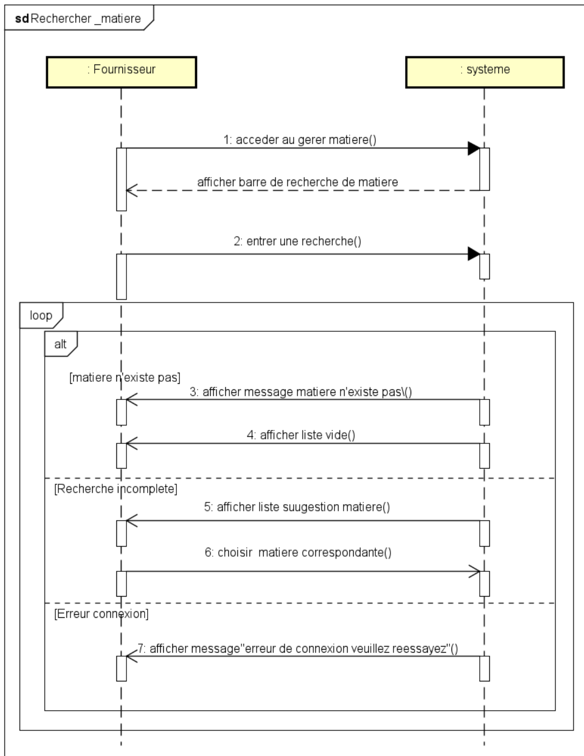
Figure 63 Diagramme de séquence rechercher matière
