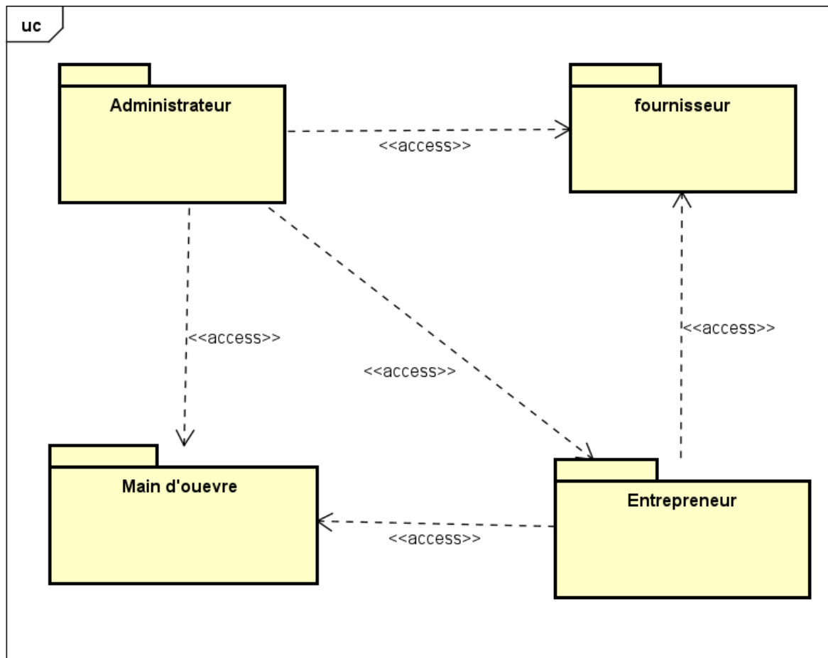
Figure 3 Diagramme du package
