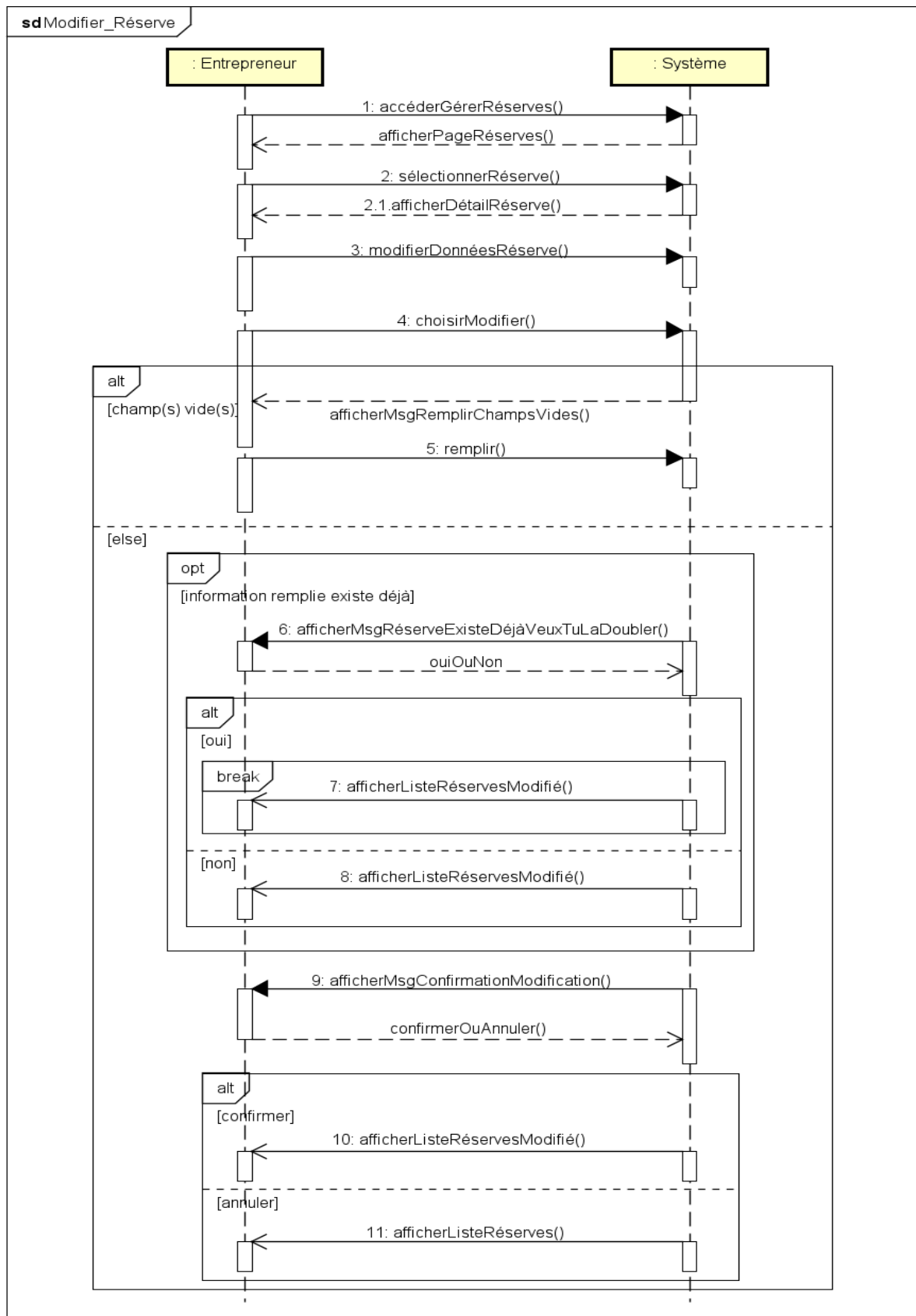
Figure 40 Diagramme de séquence de modifier réserve
