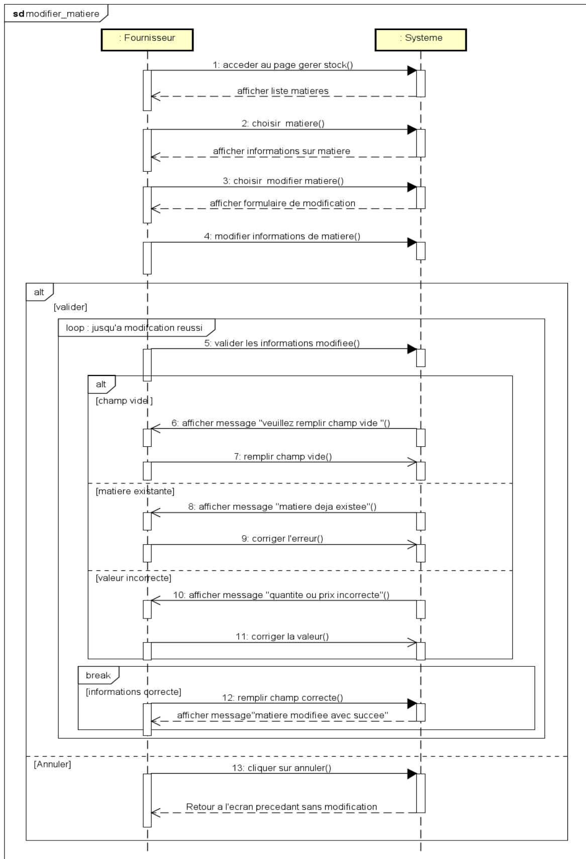
Figure 61 Diagramme de séquence de modifier matière
