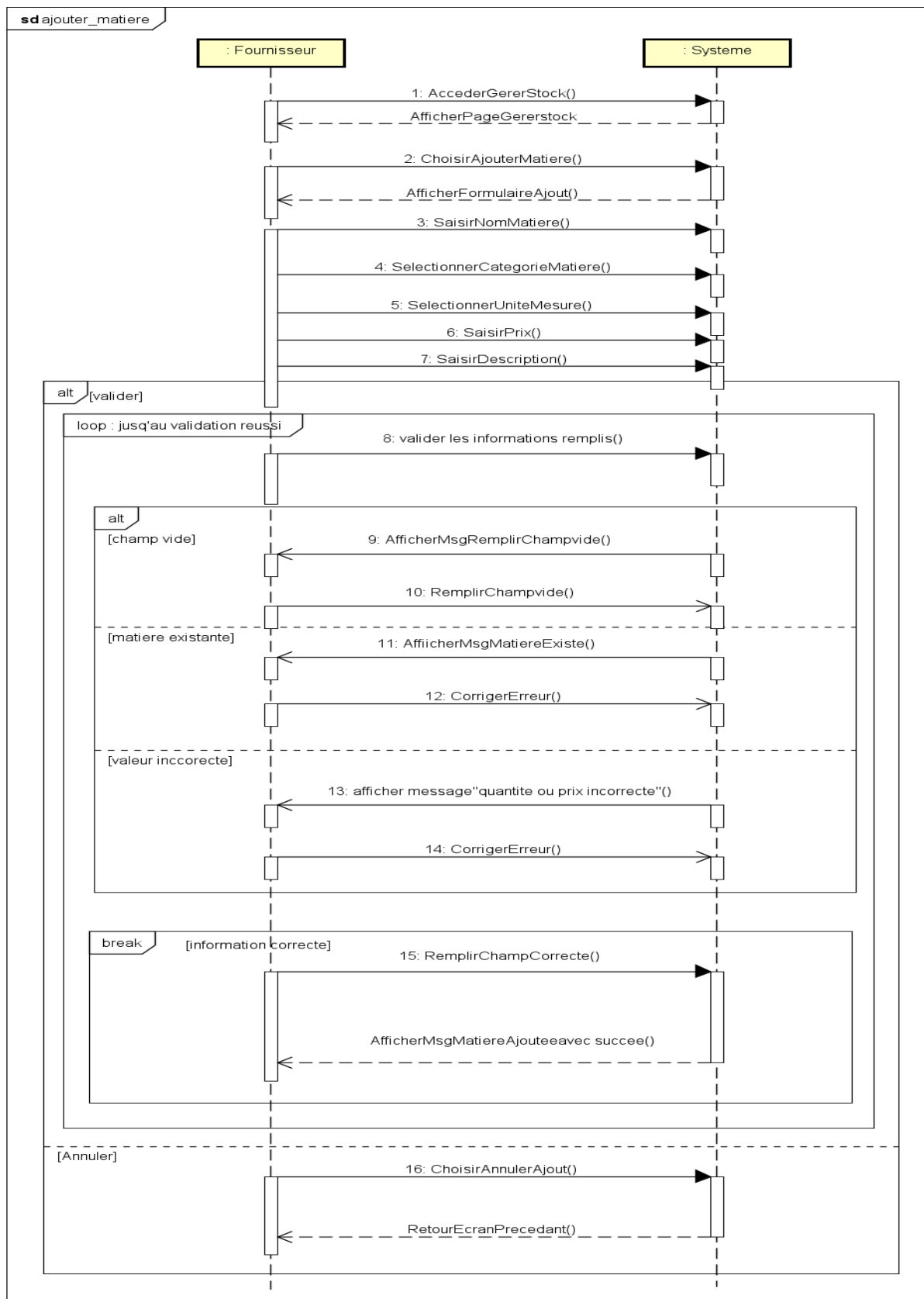
Figure 60 Diagramme de séquence ajouter matiere
