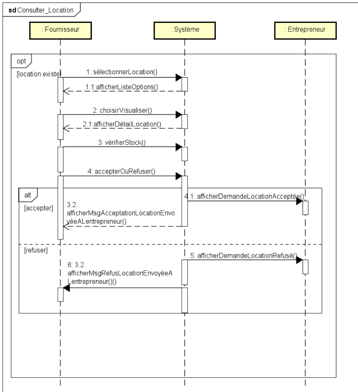
Figure 70 Diagramme de séquence de consulter location
