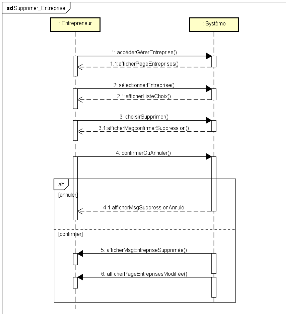
Figure 51 Diagramme de séquence de supprimer entreprise
