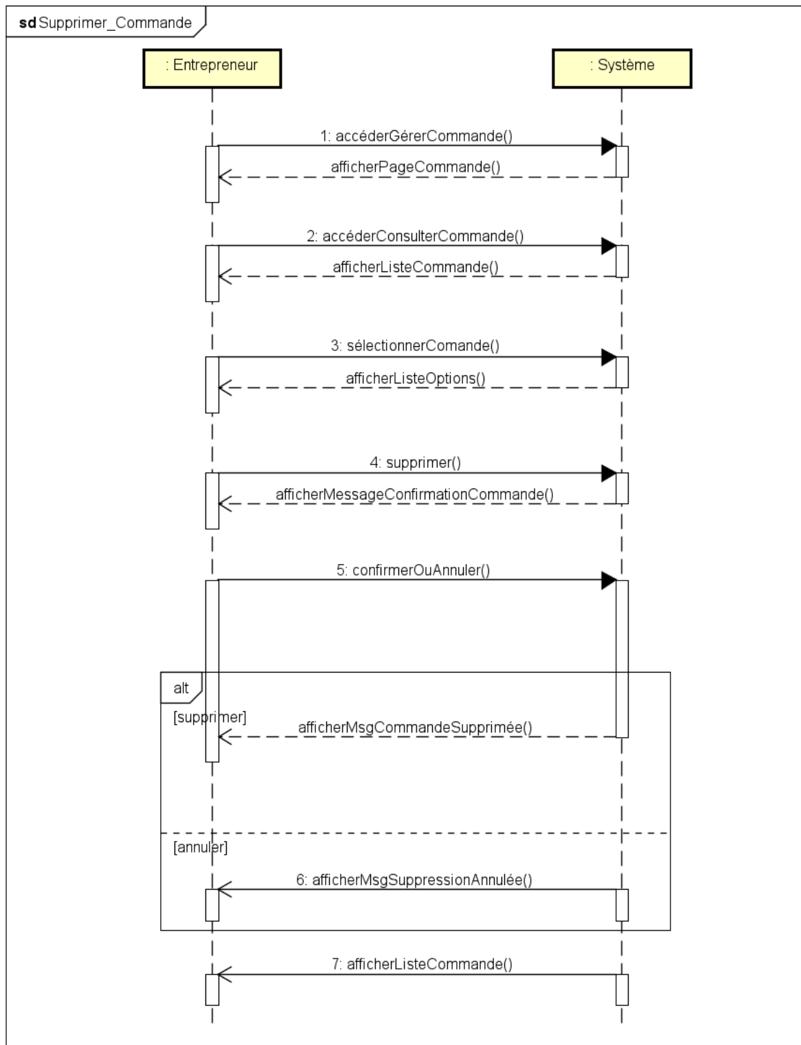
Figure 25 Diagramme de séquence de supprimer commande
