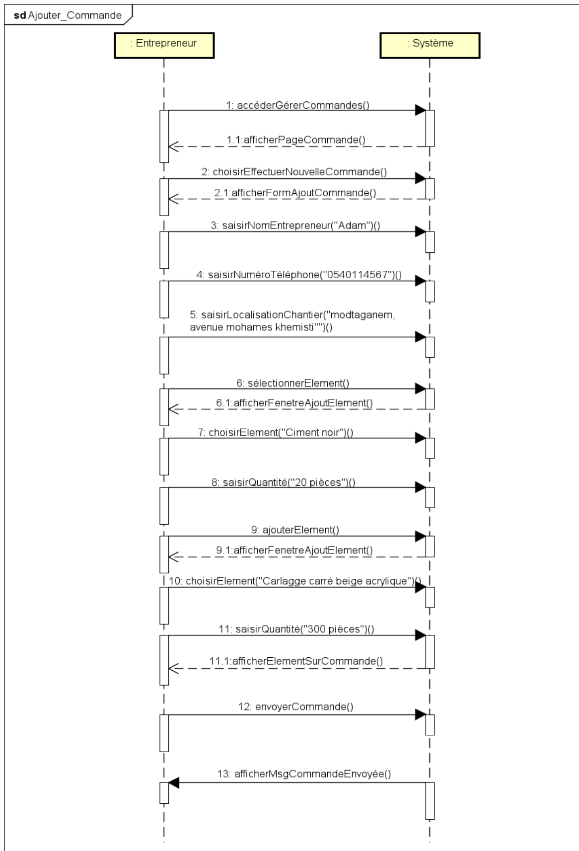
Figure 16 Diagramme de test de séquence ajouter commande
