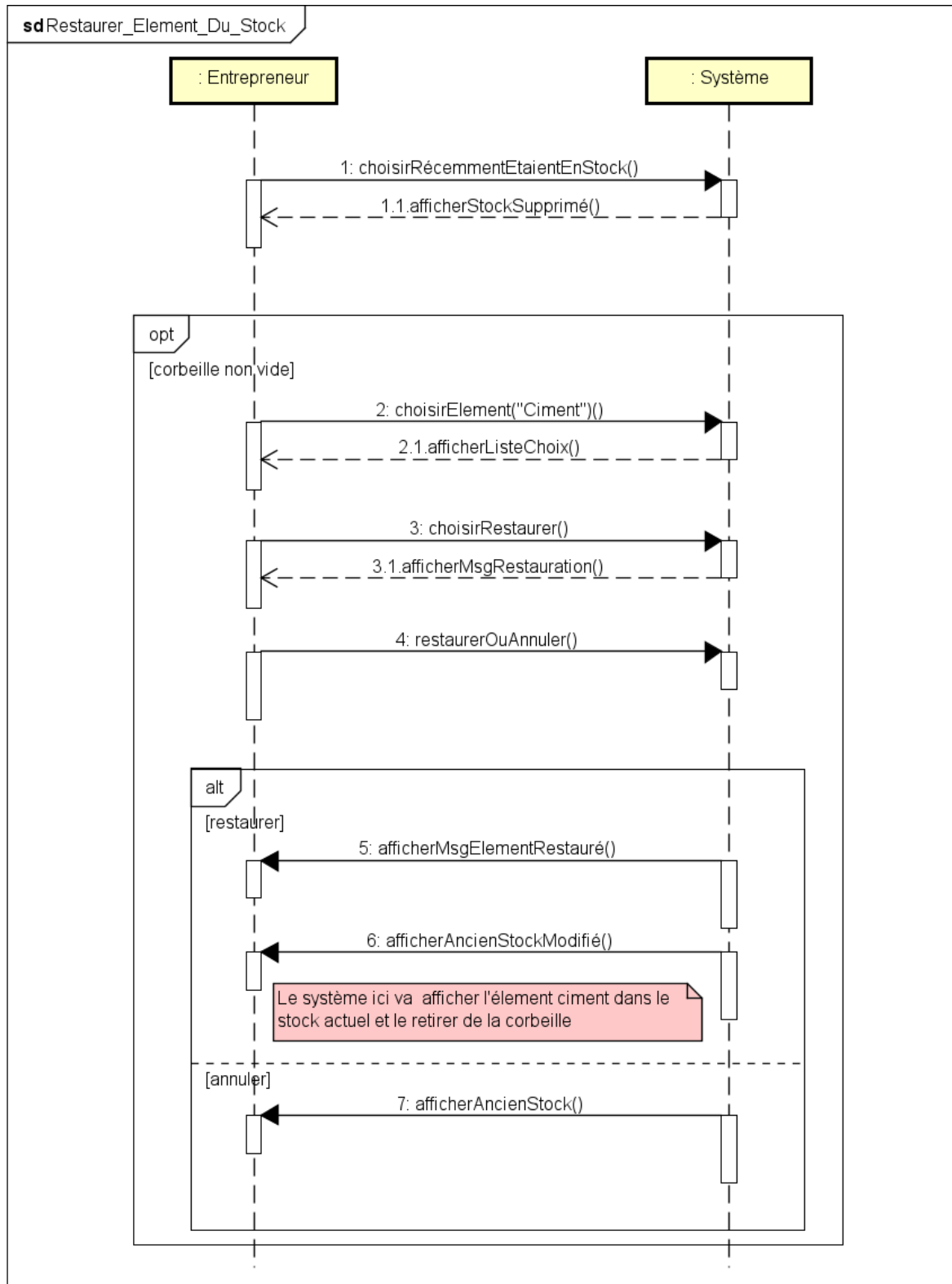
Figure 100 Diagramme de test de séquence restaurer élément du stock
