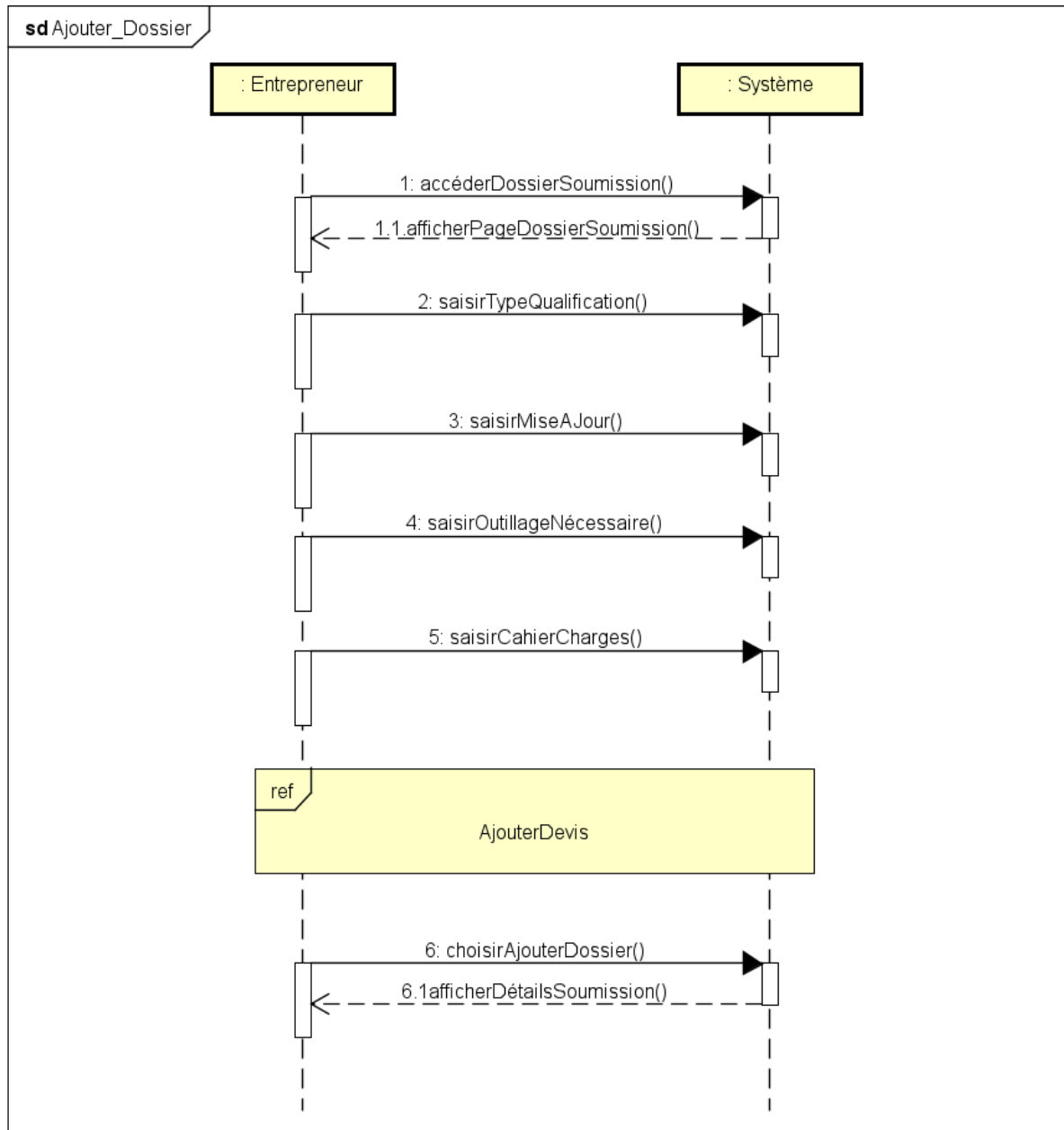
Figure 43 Diagramme de séquence d'ajouter un dossier de soumission
