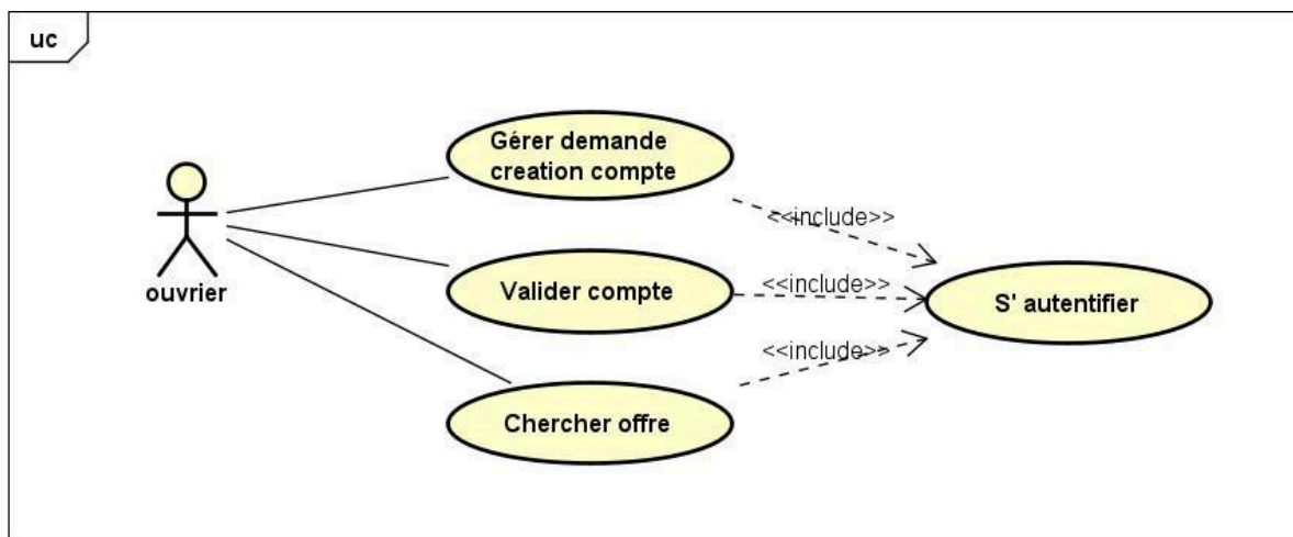
Figure 7 Diagramme de cas d'utilisation du package ouvrier
