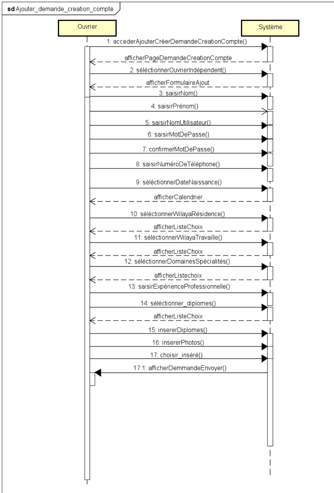
Figure 83 Diagramme de séquence Ajouter demande création compte ouvrier indépendant
