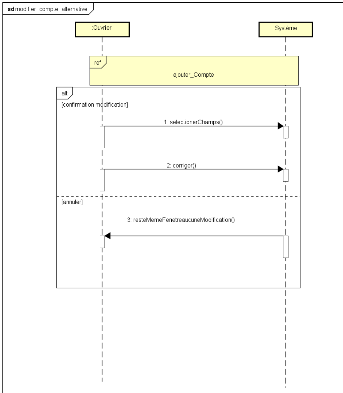
Figure 88 Diagramme de séquence de modifier demande création compte alternatif
