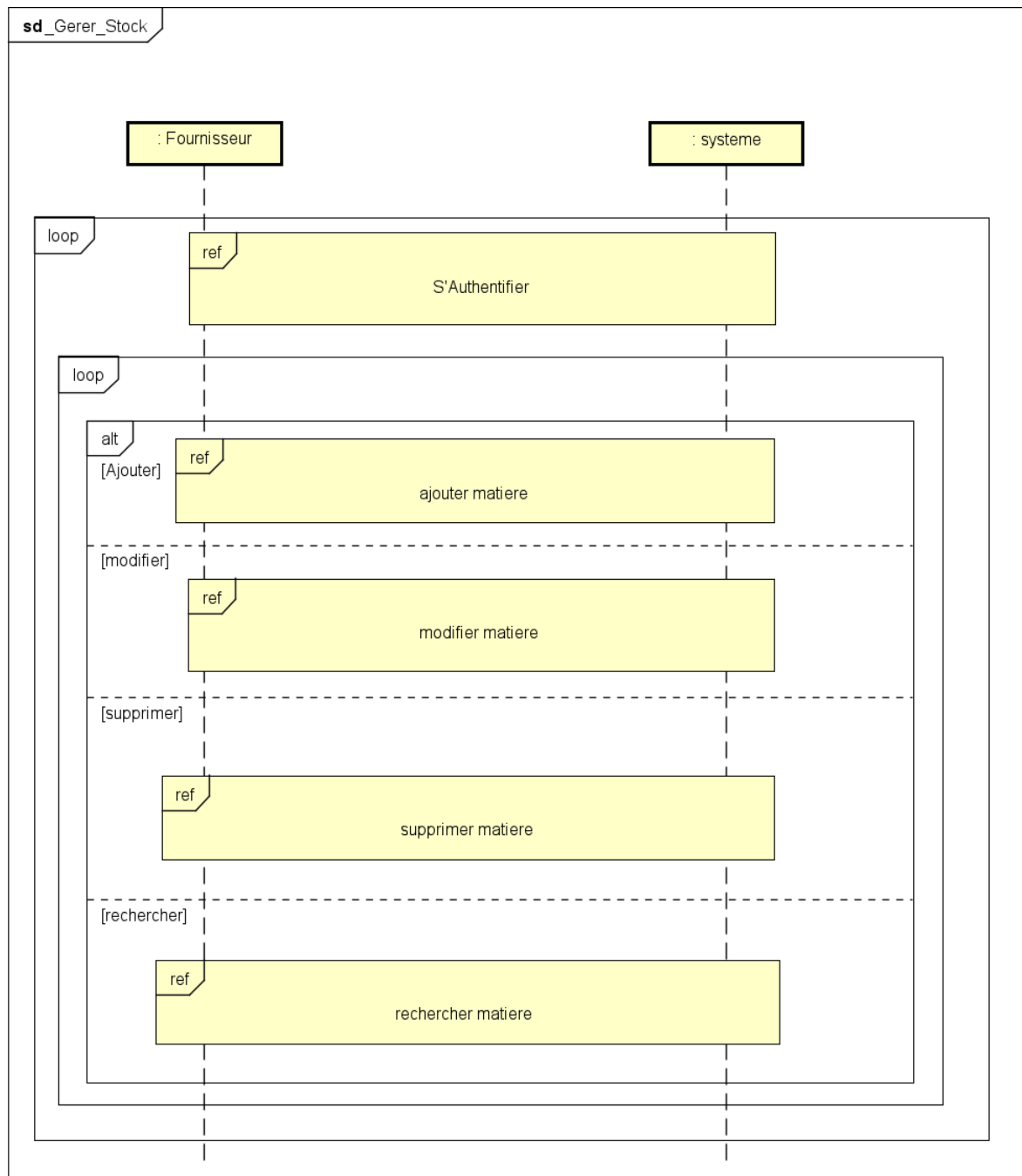
Figure 59 Diagramme de séquence de gerer stock
