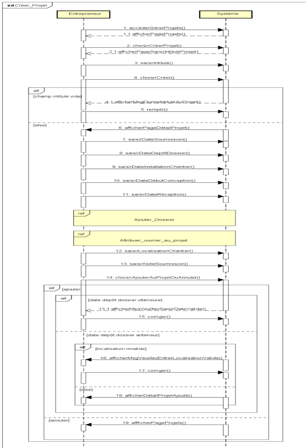
Figure 46 Diagramme de séquence de créer projet
