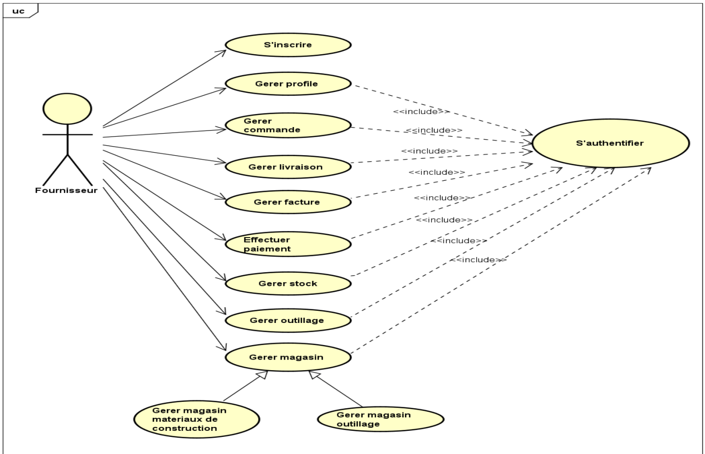
Figure 6 Diagramme de cas d'utilisation du package fournisseur
