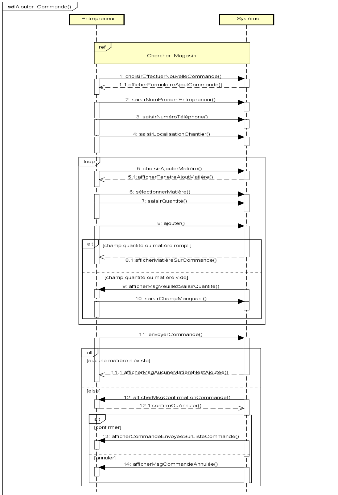
Figure 26 Diagramme de séquence d'ajouter commande
