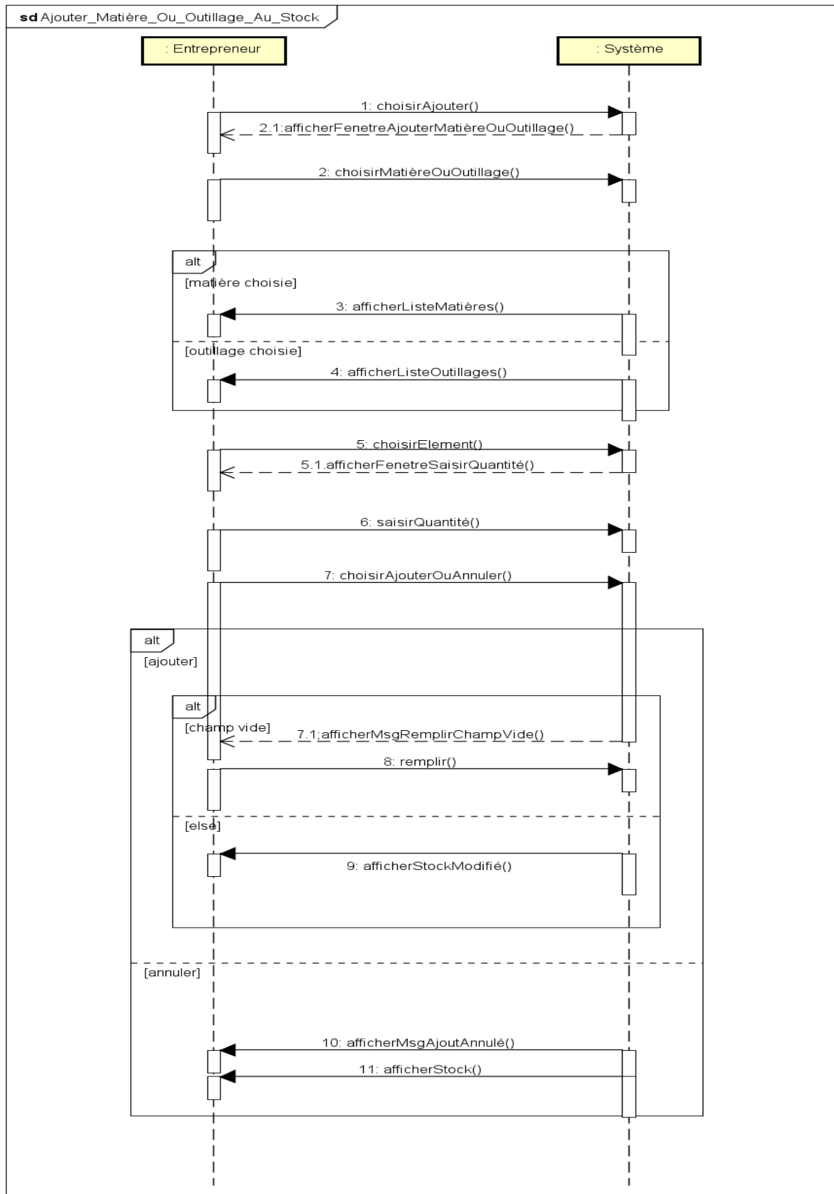
Figure 9 Diagramme de séquence d'ajout de matières ou outillages au stock
