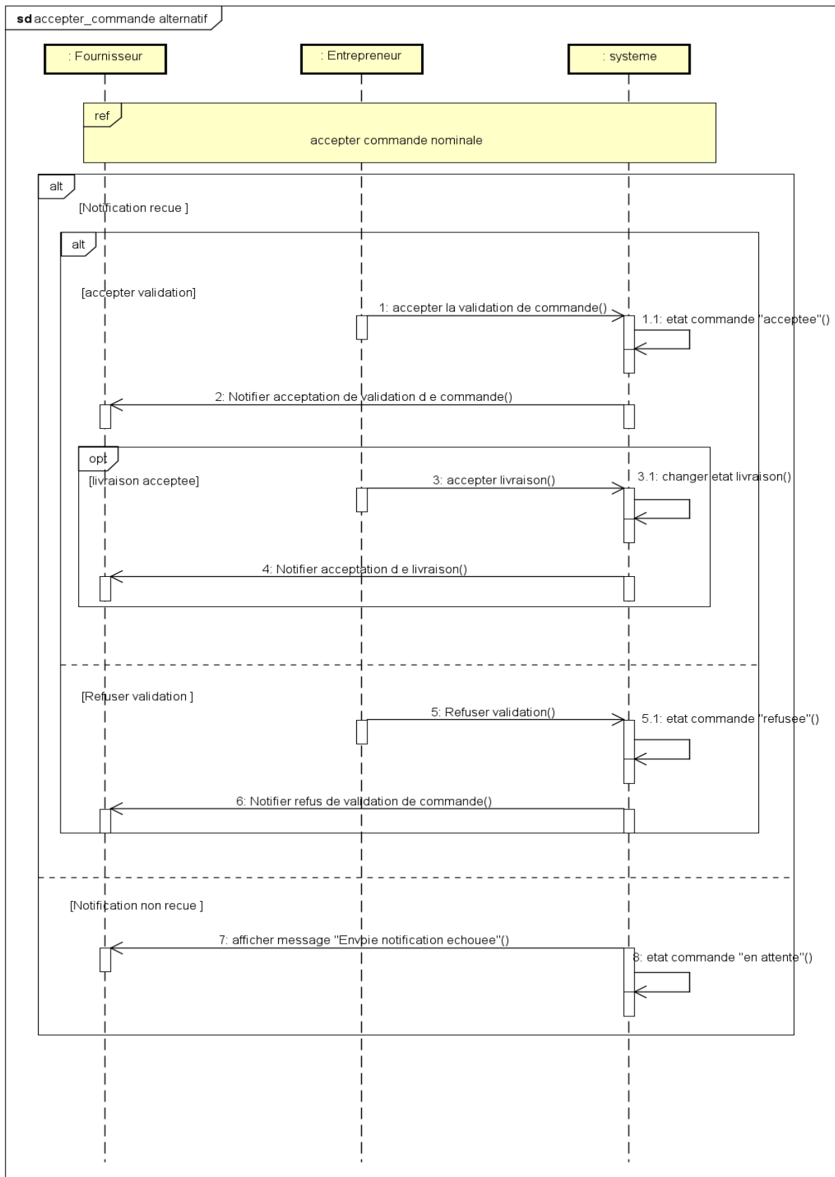
Figure 73 Diagramme de séquence accepter commande alternatif
